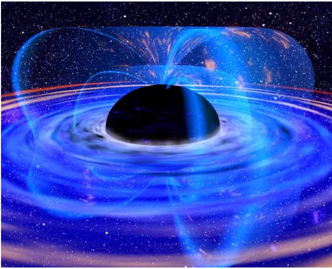
الشكل (17) تصور لثقب أسود دوّار
