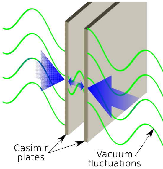
الشكل (19) تولد طاقة كازيمير الفراغية بين لوحين موصلين متعادلين
