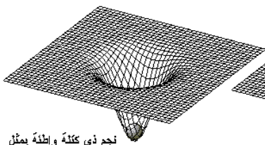
نجم ذي كتلة واطئة يمثل حفرة بسيطة في الزمكان
