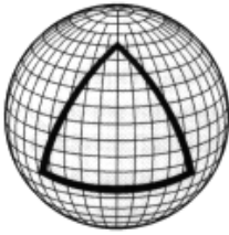
هندسة لا إقليدية مغلقة
