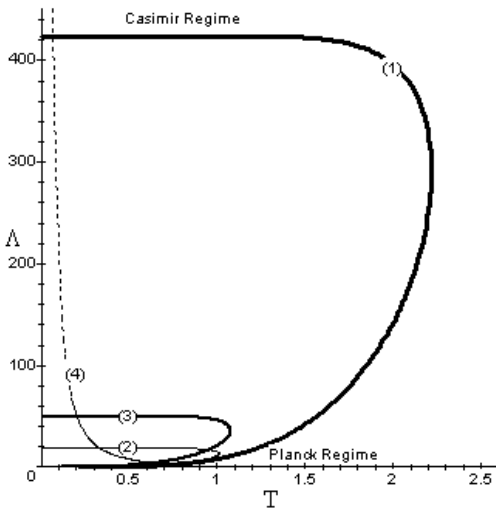
الشكل (28) تغير قيمة الثابت الكوني مع درجة حرارة الكون لمجالات كمومية متعددة في فضاء أينشتاين
