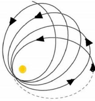
زحزحة حضيض الكواكب
