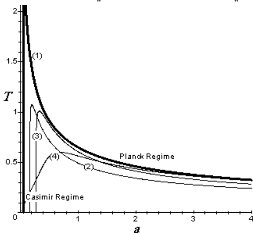
الشكل (27) تغير نصف قطر الكون مع درجة حرارته لمجالات كمومية متعددة في فضاء أينشتاين
