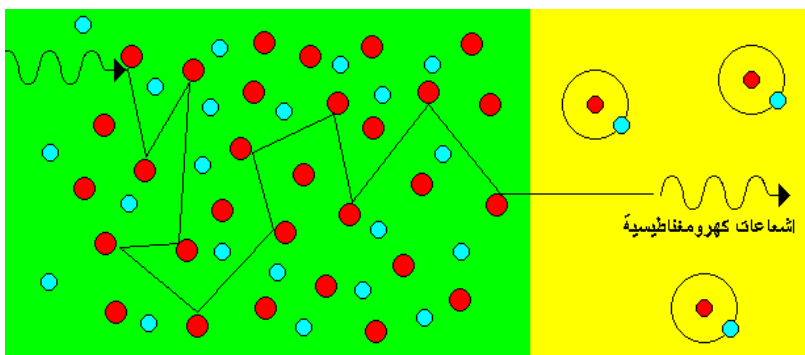
ذرات الهيدروجين والهيليوم المتأينة
