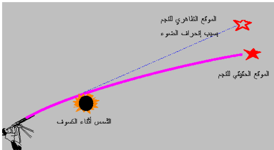
الشكل (14) إنحراف الضوء بتأثير الجاذبية
