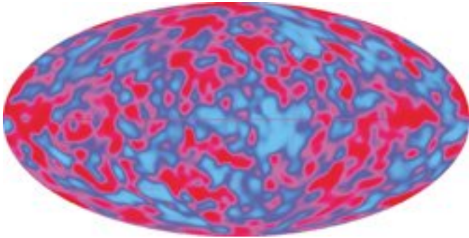
الشكل (21) التوزيع الزاوي للخلفية المايكروية الكونية بحسب نتائج كوب
