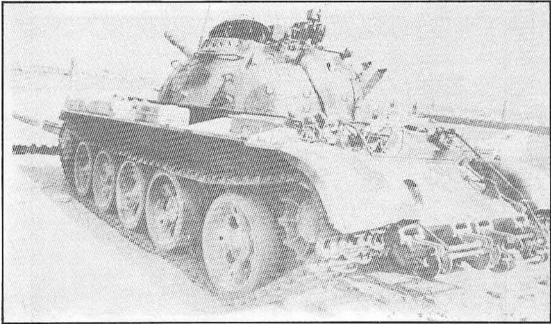
دبابة من نوع «تي 55» غنمتها القوات المسلحة الملكية وهي صالحة للاستعمال (يناير 1984) من مميزات هذه الدبابة تتوفر على مدفع 100 مم ورشاشتين وعلى الأشعة مائح الحمراء التي تمكنها من العمل ليلا. وتستطيع السير في الماء بواسطة مراوح تشبه مراوح السفينة.
