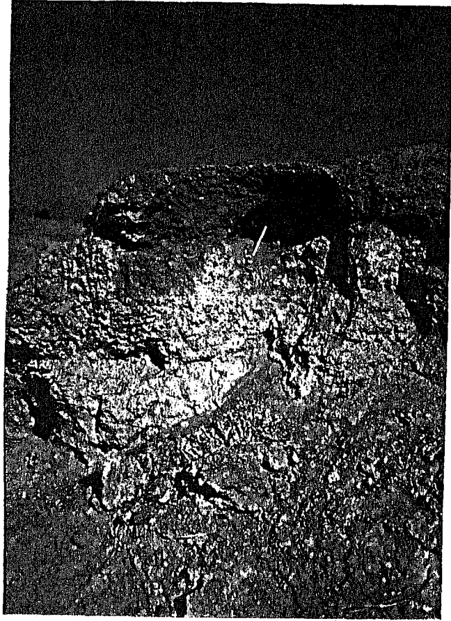
صورة رقم (١١) توضح طبقات الطفل المتباينة والتي تتوزع وسط وشمال منطقة الدراسة .
