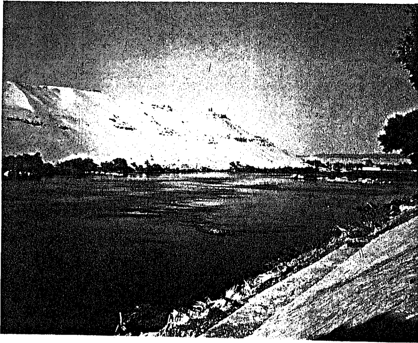
صورة ( ٤٨ ) يوضح الجزء الأيمن منها الجانب المقعر والذي تم تكسيته - والجزء الأيسر منها يوضح الجانب المحدب لمنعطف قبة الهوا . ( أتجاه النظر صوب الشمال الغربي )
