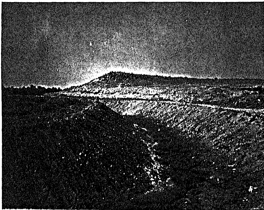
صورة (٤٤) توضح السهل الفيضي حيث لا يزيد عن ٢ كم عند نجع سيدى الشيخ مصطفى عبد السلام ذلك على الجانب الايسر للصورة ويوضح الجانب الايمن الحافة الرئيسية والتي تطل على نهاية السهل الفيضي . اسفل الصورة يظهر مصرف السيل ( اتجاه النظر نحو الشمال الشرقى )
