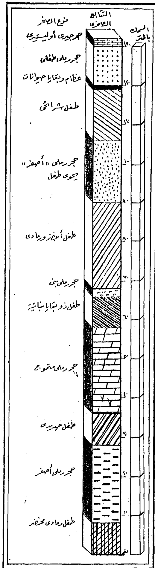
المصدر: (Beadnell) شكل (٦)
