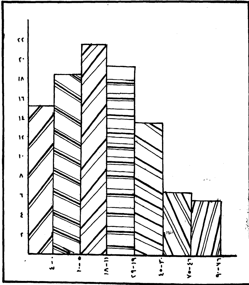
شكل (٢٧) فئات زوايا الانحدار منطقة الدراسة
