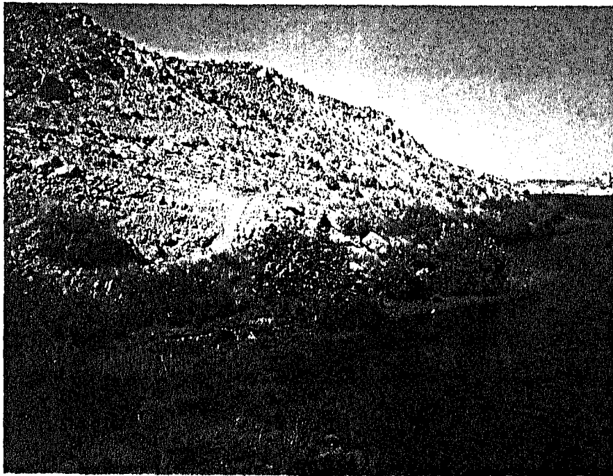
صورة (٢٤) الجانب الشرقى لجزيرة هيسا (اتجاه النظر صوب الجنوب الشرقى)
