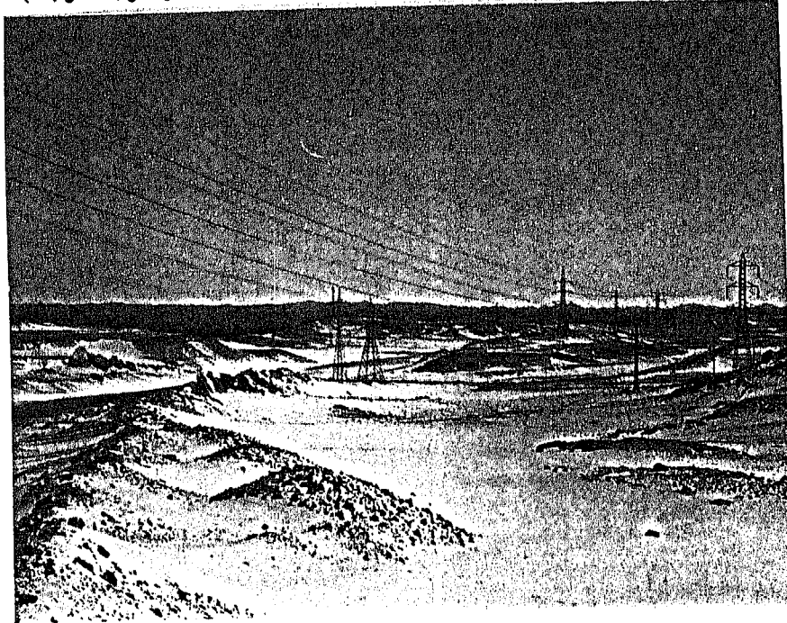
صورة رقم (١٦) توضح الاسطح الحصوية المختلطة بالرمال الخشنة منظر متكرر غرب النيل (اتجاه النظر صوب الجنوب الشرقي )
