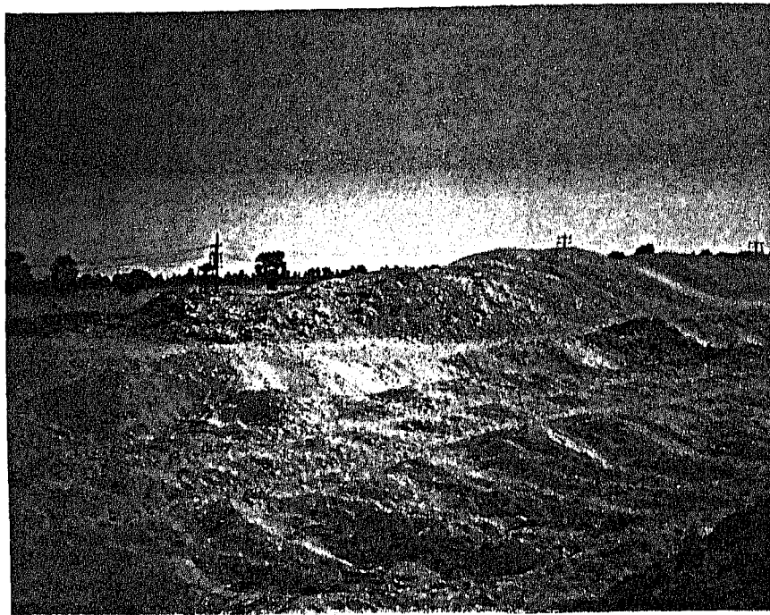
صورة (٤٣) توضح الجزر الرملية والتي تمثل الخطوط الفاصلة بين تربة السهل الفيضي القديم وتربة الاودية الجافة ( شرق كلابشة الجديدة ) منظر متكرر شرق الشطب ، وشرق السلسلة . ( اتجاه النظر صوب الشرق )
