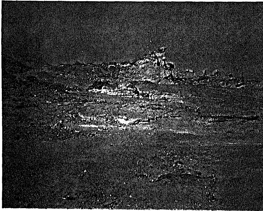
صورة رقم (٥٧) المنحدرات شبه السلمية شمال الكاجوج . ( اتجاه النظر صوب الشمال الغربي )
