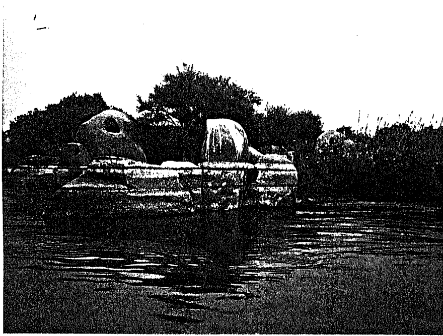
صورة (٣٢) توضح ظاهرة طلاء الصحراء على صخور الجندل الأول وتحويل اللون الوردى إلى لون داكن. (اتجاه النظر صوب الغرب)
