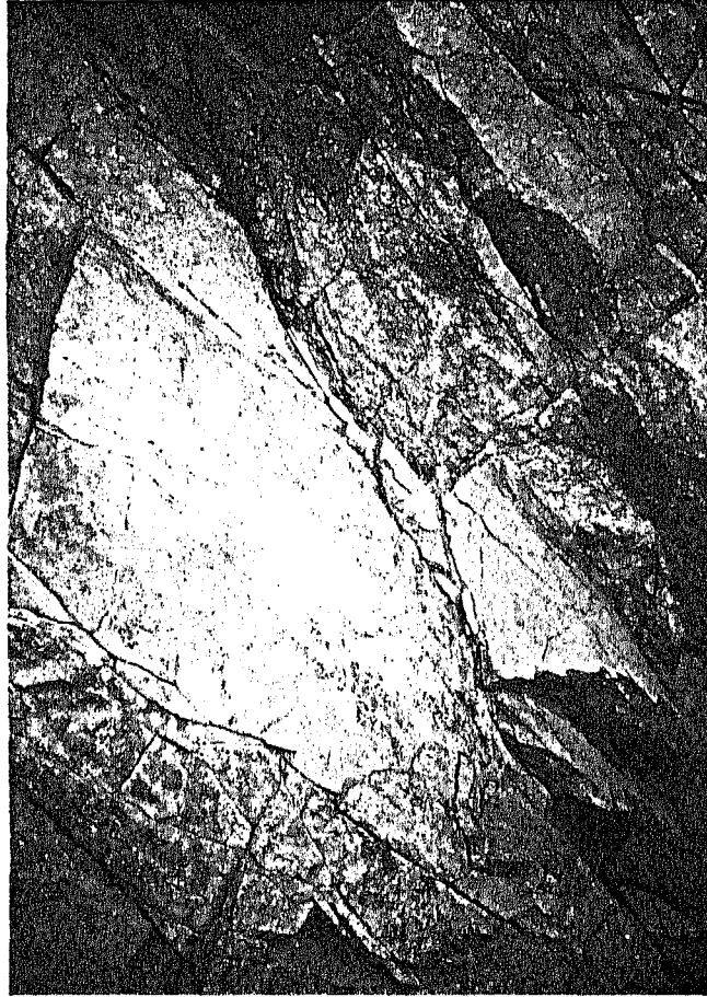
صورة (٢٠) توضح الإنكسارات في الصخور النارية . ( اتجاه النظر صوب الشرق )
