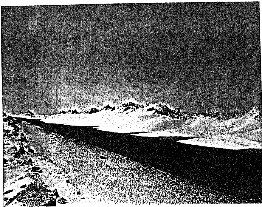
صورة رقم (١٤) توضح الغطاءات الرملية التي تنقلها الرياح وتغطي أجزاء من الطريق غرب النيل وهي ظاهرة متكررة من شمال أسوان وحتى جنوب ادفو.(اتجاه النظر صوب الجنوب الغربى )
