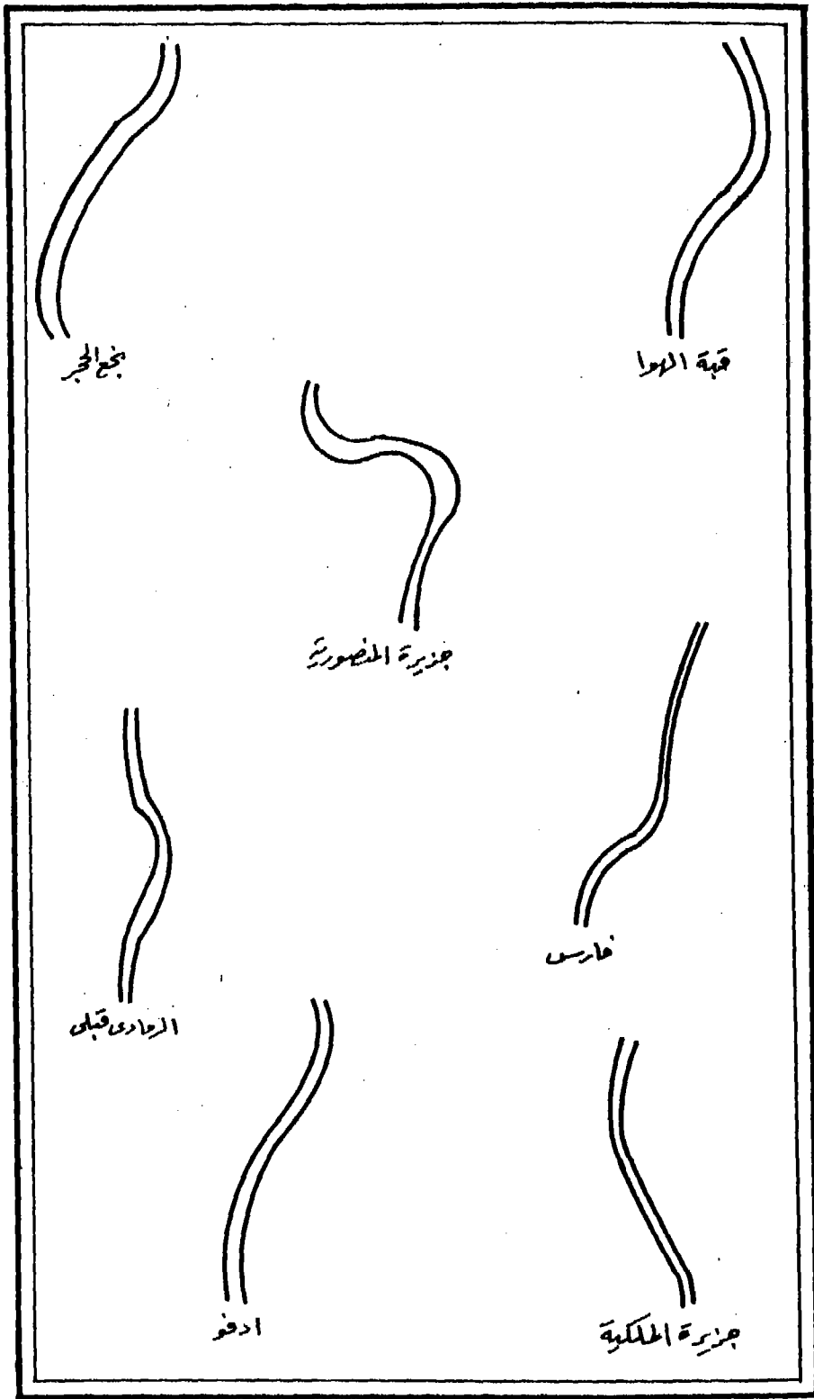
شكل (١٢) أشكال المنعطفات النهرية في منطقة الدراسة .
