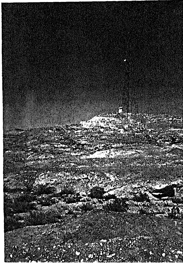
صورة رقم (٥٦) توضح المنحدرات شبه السلمية في منطقة جعفر الصادق . ( اتجاه النظر صوب الشمال الغربي )
