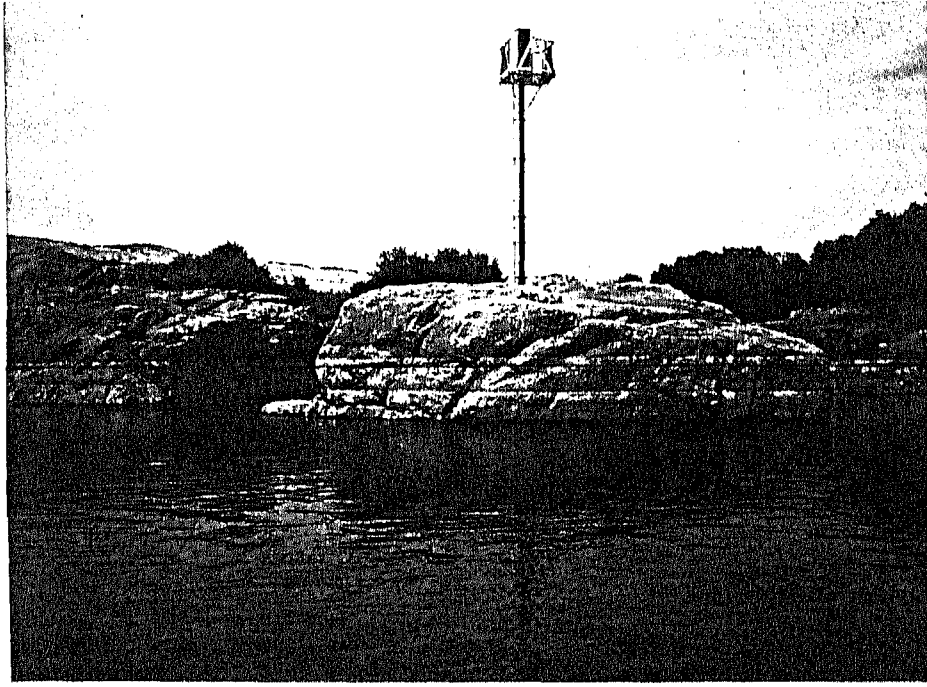
صورة (٧) توضح الصخور النارية المكونة للجزر الصخرية بوسط المجرى امام أسوان ( ا تجاه النظر صوب الغرب)
