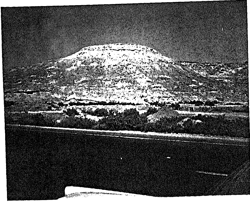
صورة رقم (٥٤) منحدرات الجروف المقعرة عند مصب وادي عباد . ( اتجاه النظر صوب الشمال الشرقى )
