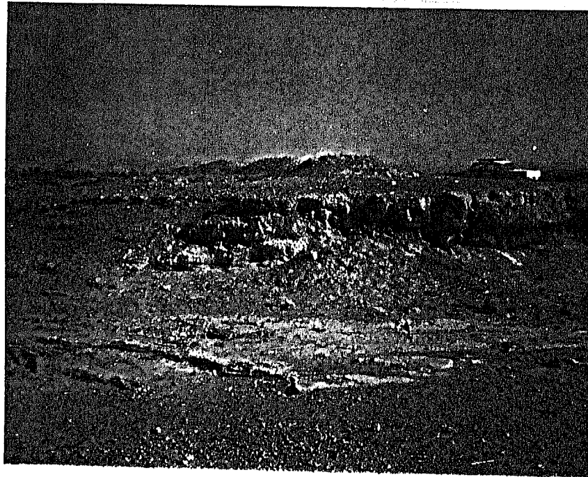
صورة رقم (٦١) توضح المصاطب الرسوبية - ظاهرة تنتشر عند مصبات الاودية. ( اتجاه النظر الشمال الغربي )
