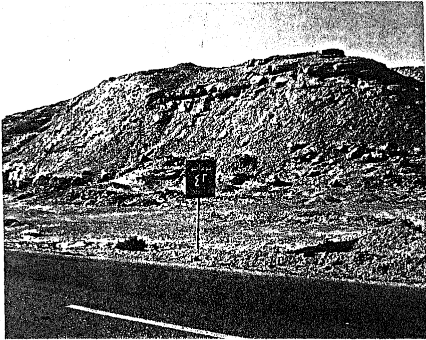
صورة رقم (٥٥) منحدرات الجروف جنوب مصب وادي السراج ( شمال كوم أمبو ) . ( اتجاه النظر الشمال الغربى )
