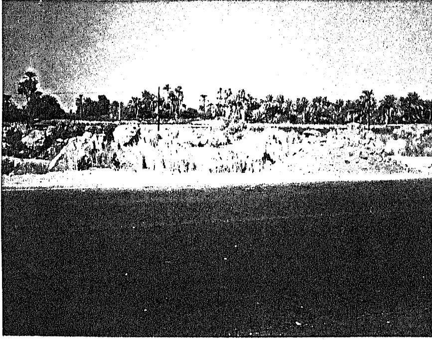
صورة (٢٨) الجلاميد المكورة جنوب الرديسية. ( اتجاه النظر صوب الشمال الشرقى ) .
