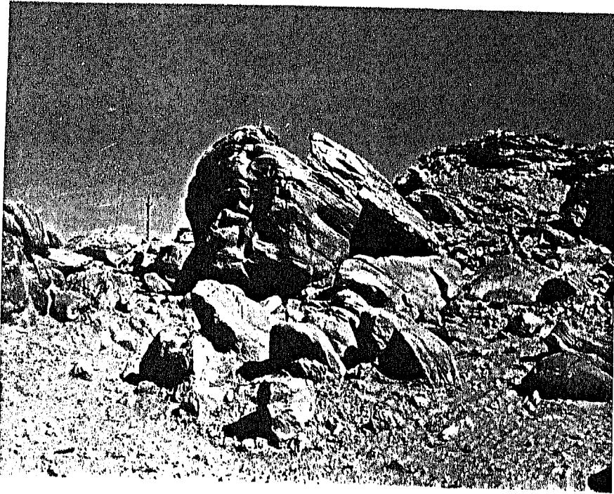
صورة (٢٩) تفلق الصخور نتيجة فعل الحرارة ويلاحظ الجلاميد المكورة اسفل الصورة - جنوب نجم السيد سعيد ( اتجاه النظر صوب الغرب ) .
