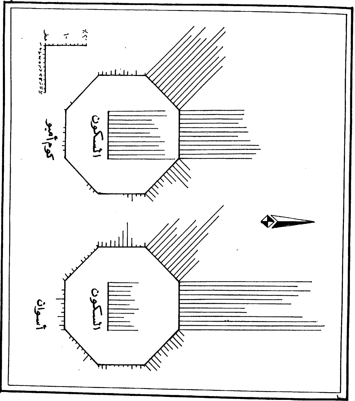
شكل "١٣" اتجاهات ونسب جهوب الرياح في محطتي كوم أمرو وأسوان
