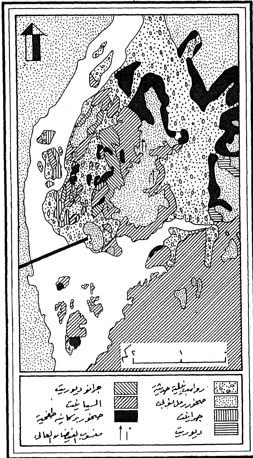
شكل (٣) المصدر: (said, 1962)
