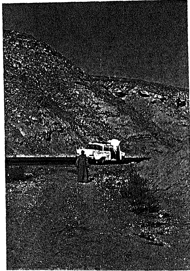
صورة رقم (٥٣) المنحدرات المحدبة - المقعرة على جوانب مصب وادي السراج . ( اتجاه النظر الشمال الغربي )
