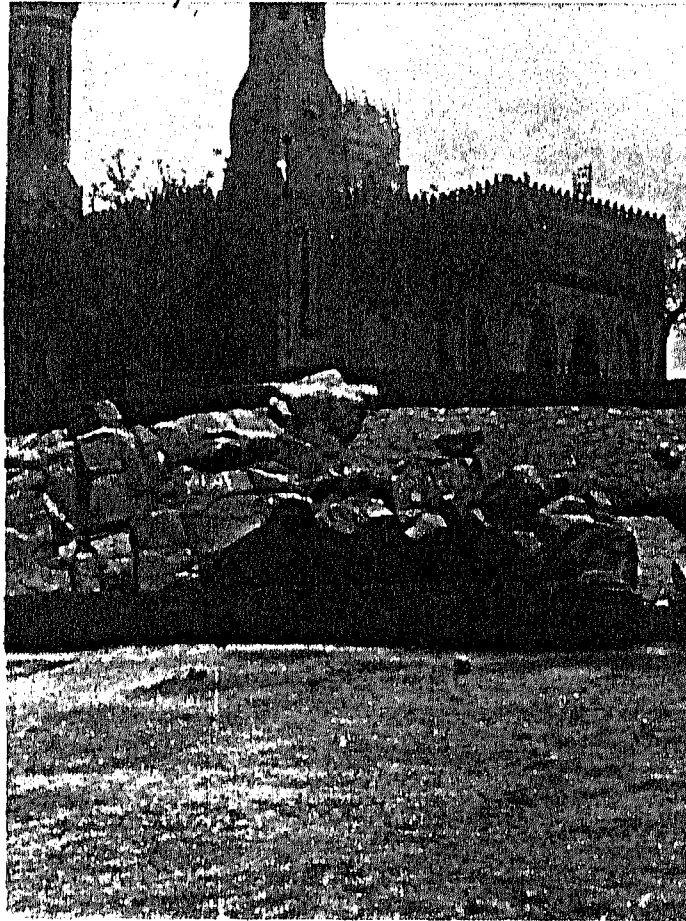
صورة (٧) توضح الصخور النارية المكونة للجزر الصخرية بوسط المجرى امام أسوان ( ا تجاه النظر صوب الغرب)
