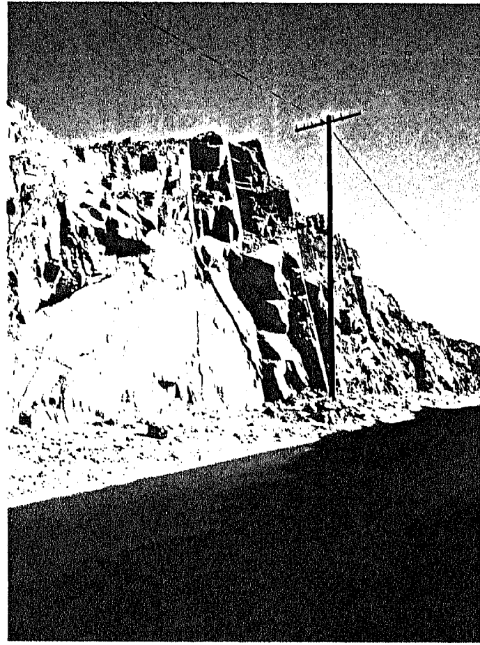
صورة رقم (٥) توضح مكاشف من صخور النيس والشست شرق السد العالى (اتجاه النظر صوب الشمال الشرقى )
