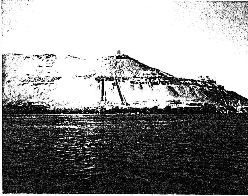
صورة رقم (٩) توضح كتلة الحجر الرملي النوبي والتي تعلوها قبة الهوا شرق أسوان . (اتجاه النظر صوب الغرب)
