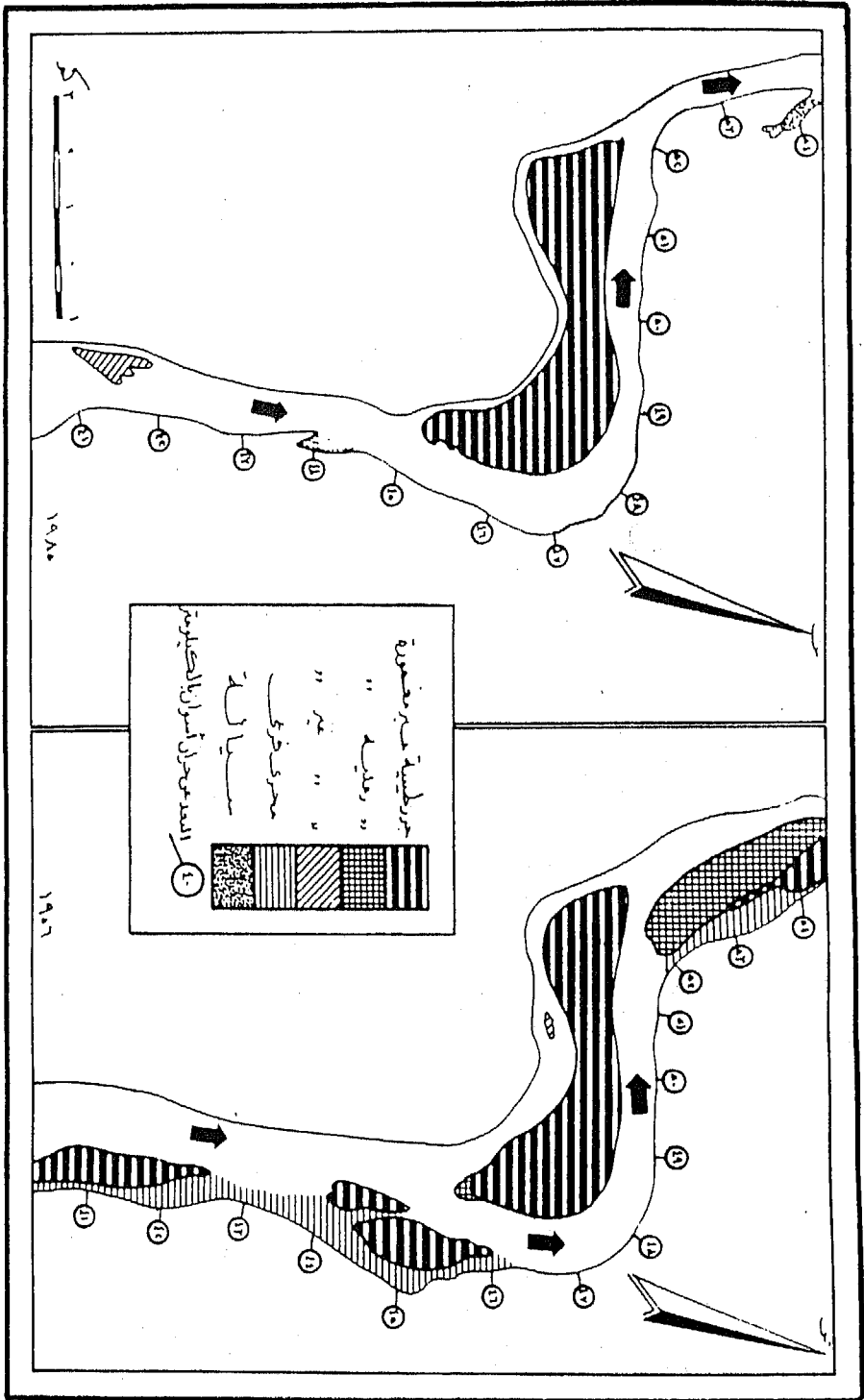
شكل (٣١) التطور الجيومورفولوجي لجزيرة المنصورة. المصدر: (نصر سالم، ١٩٩٣ ص ٨٧)
